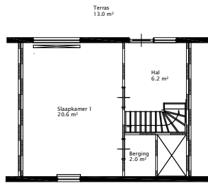
2e verdieping
